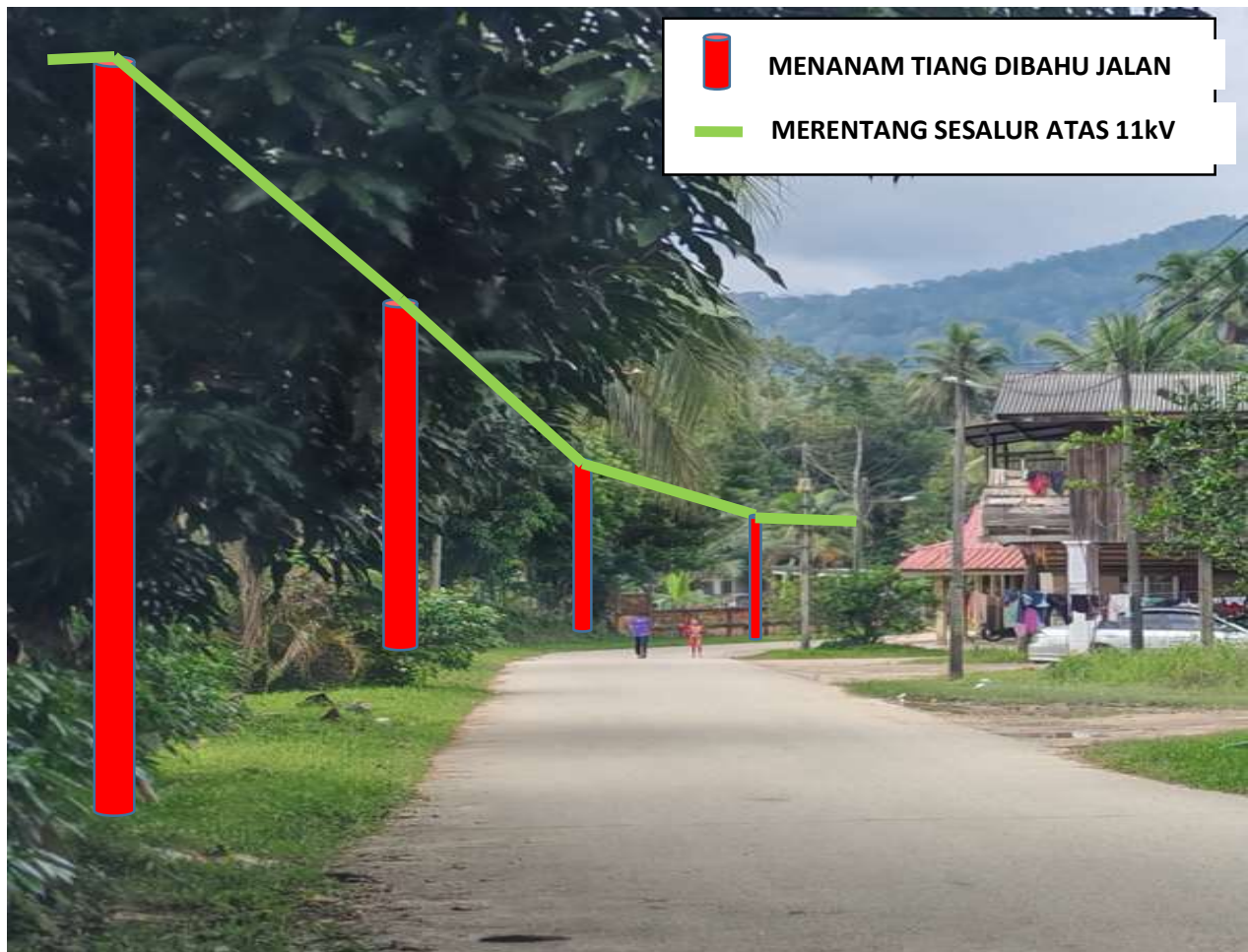
GAMBAR 5 : KAWASAN KERJA MENANAM TIANG 10M(5.0kN) DAN RENTANGAN SAVT.
