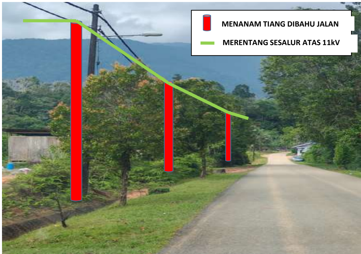
GAMBAR 4 : KAWASAN KERJA MENANAM TIANG 10M(5.0kN) DAN RENTANGAN SAVT.
