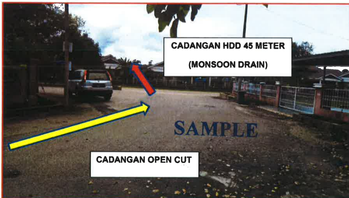
GAMBAR 4 : KAWASAN KERJA MELIBATKAN PEMOTONGAN JALAN (OPEN CUT) DAN 'HORIZONTAL DIRECTIONAL DRILLING'
