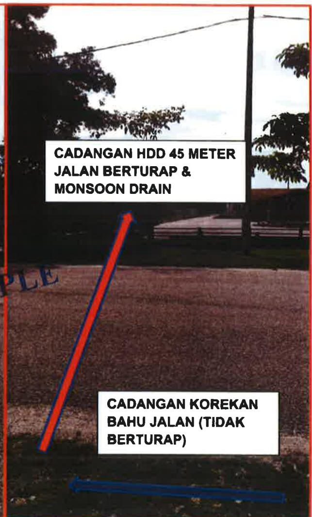
GAMBAR 8 : KAWASAN KERJA MELIBATKAN PEMOTONGAN JALAN BERTURAP DAN 'HORIZONTAL DIRECTIONAL DRILLING'
