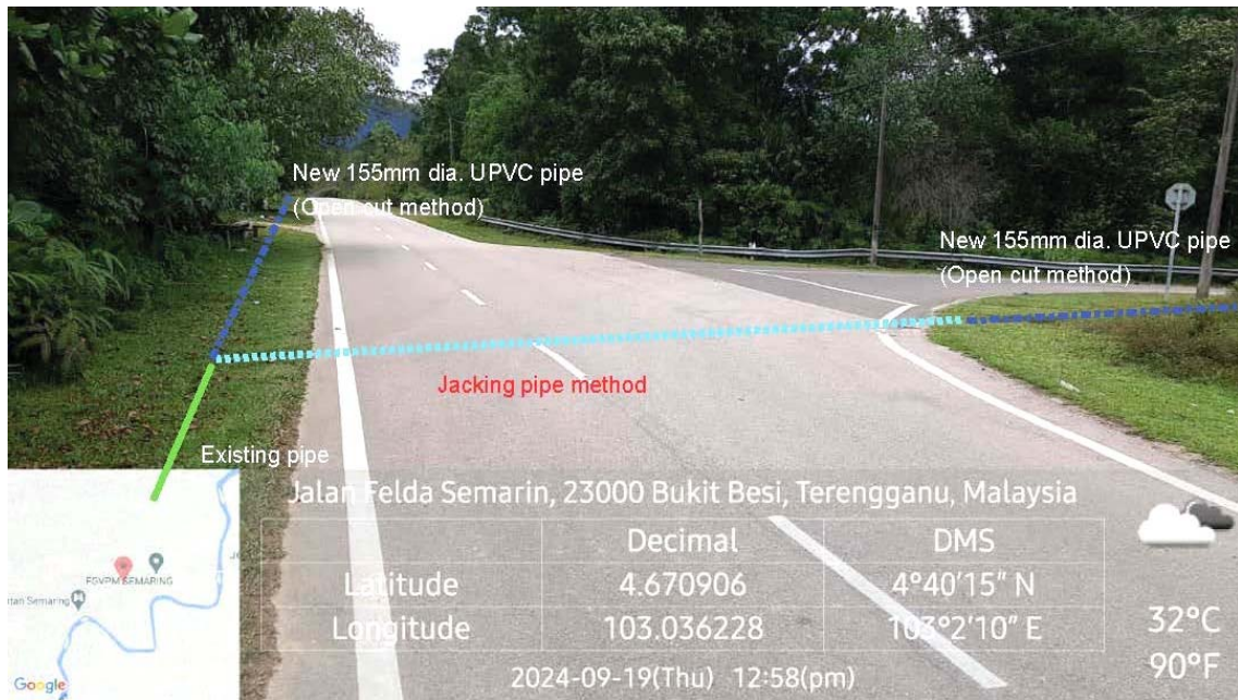
GAMBAR 3 : Kawasan 2adangan laluan paip baru dan sambungan ke paip sedia ada.
