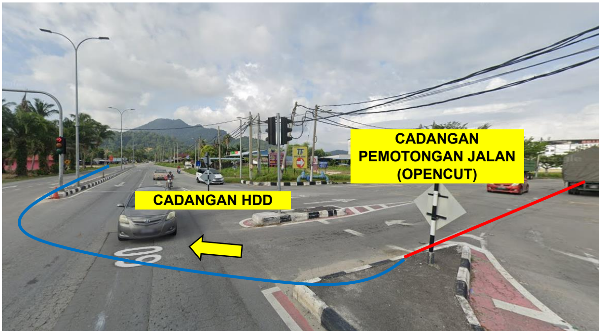
GAMBAR 6: KAWASAN KERJA MELIBATKAN PEMOTONGAN JALAN (OPENCUT) DAN 'HORIZONTAL DIRECTIONAL DRILLING'
