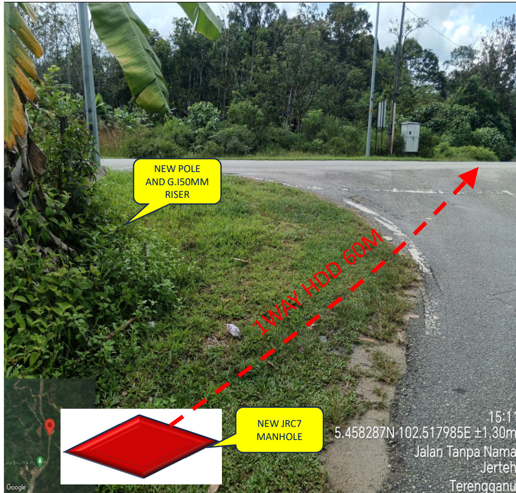
NEW 1WAY HDD JALAN TANPA NAMA KG PAK SIK KERUAK BESUT
