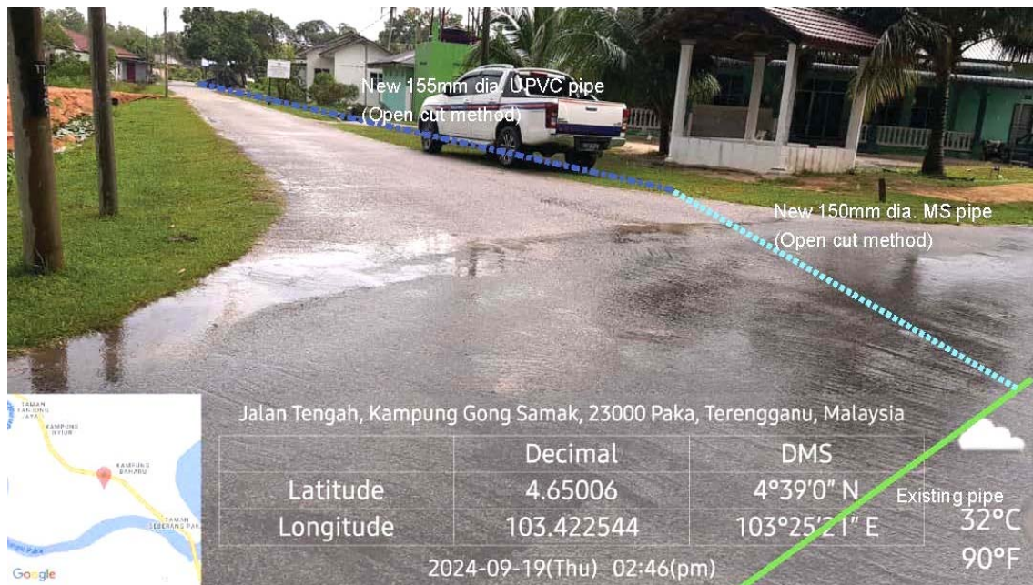
GAMBAR 3 : Kawasan adangan laluan paip baru dan sambungan ke paip sedia ada.
