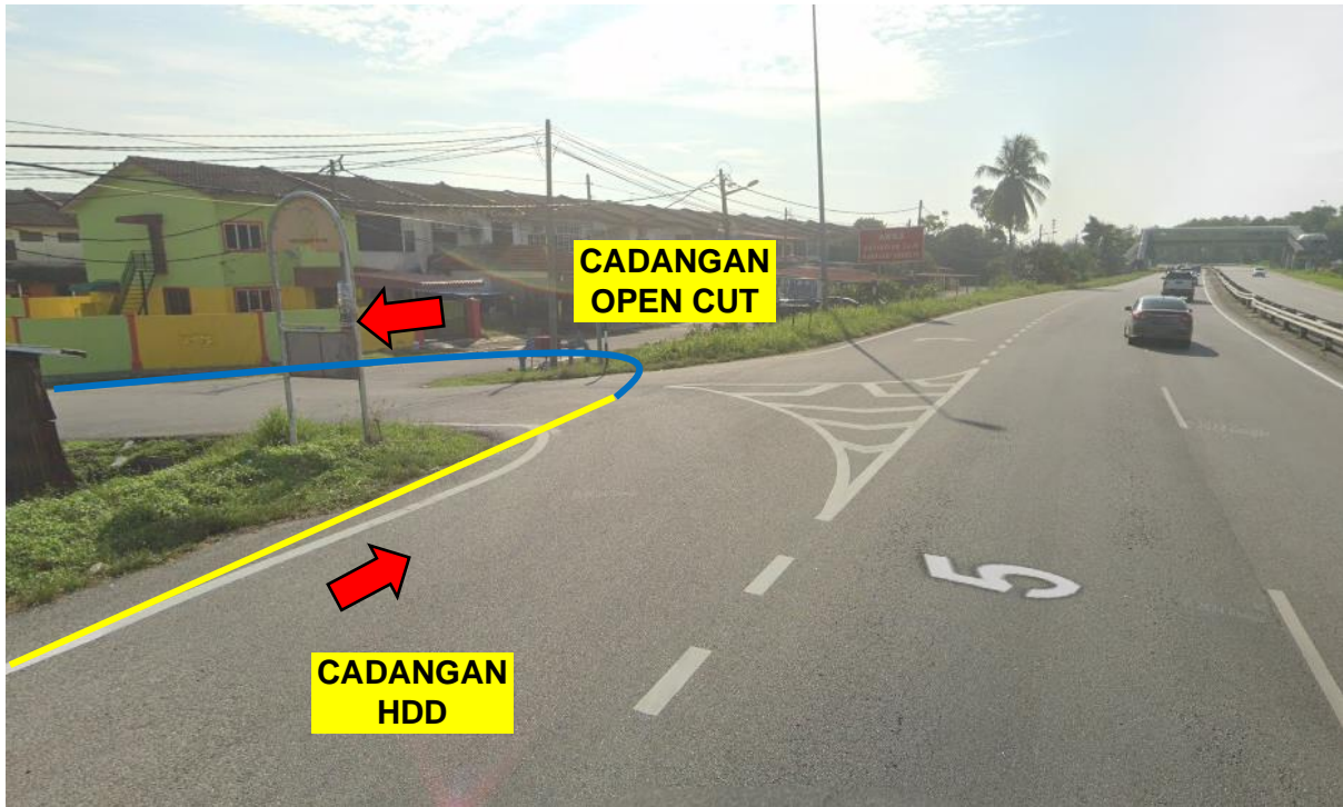
GAMBAR 3: KAWASAN KERJA MELIBATKAN 'HORIZONTAL DIRECTIONAL DRILLING' DAN PEMOTONGAN JALAN (OPEN CUT)
