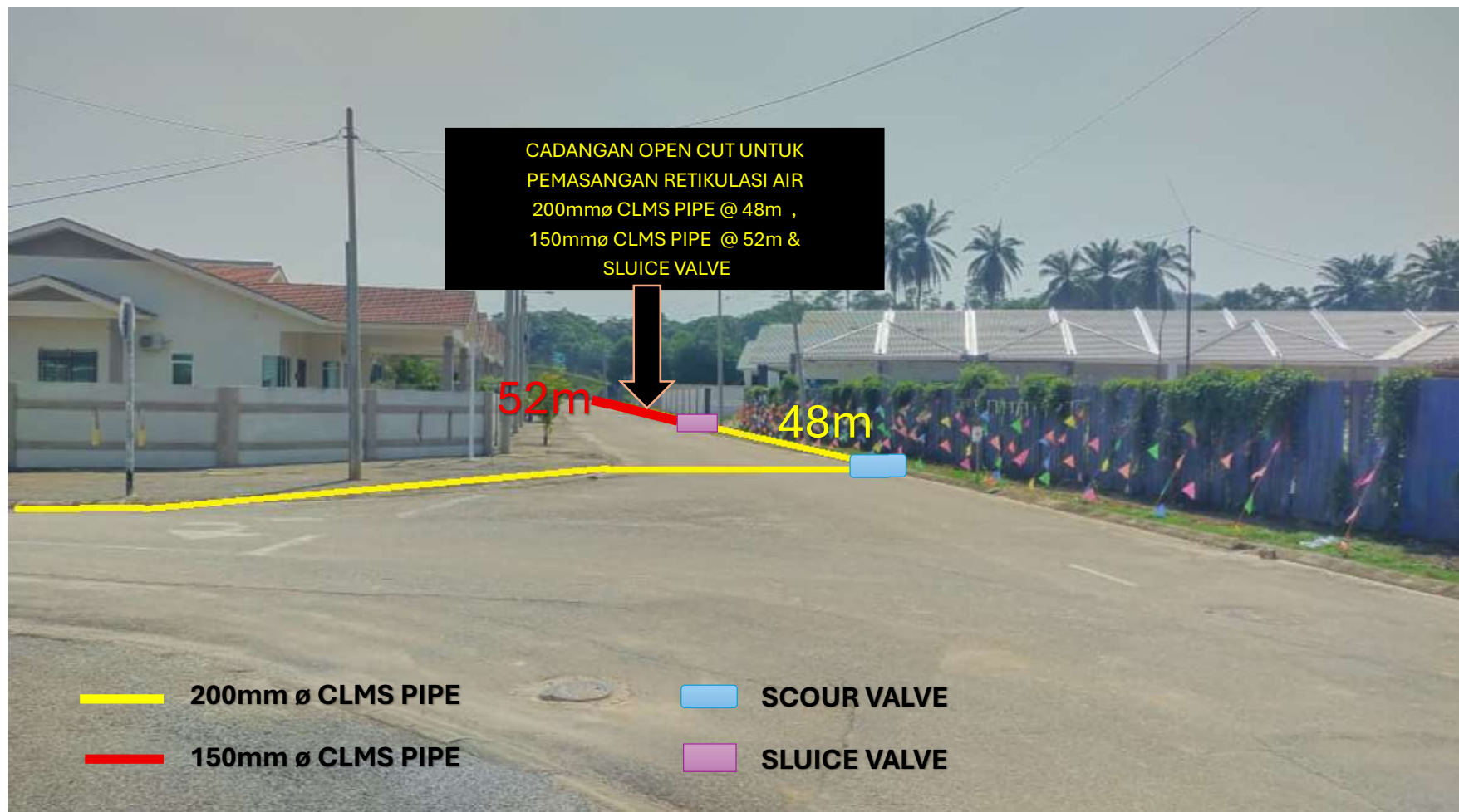
Gambar 3 : KAWASAN KERJA MELIBATKAN PEMOTONGAN JALAN (OPEN CUT) 200mmø CLMS PIPE @ 48m ,150mmø CLMS PIPE @ 52m & SLUICE VALVE
