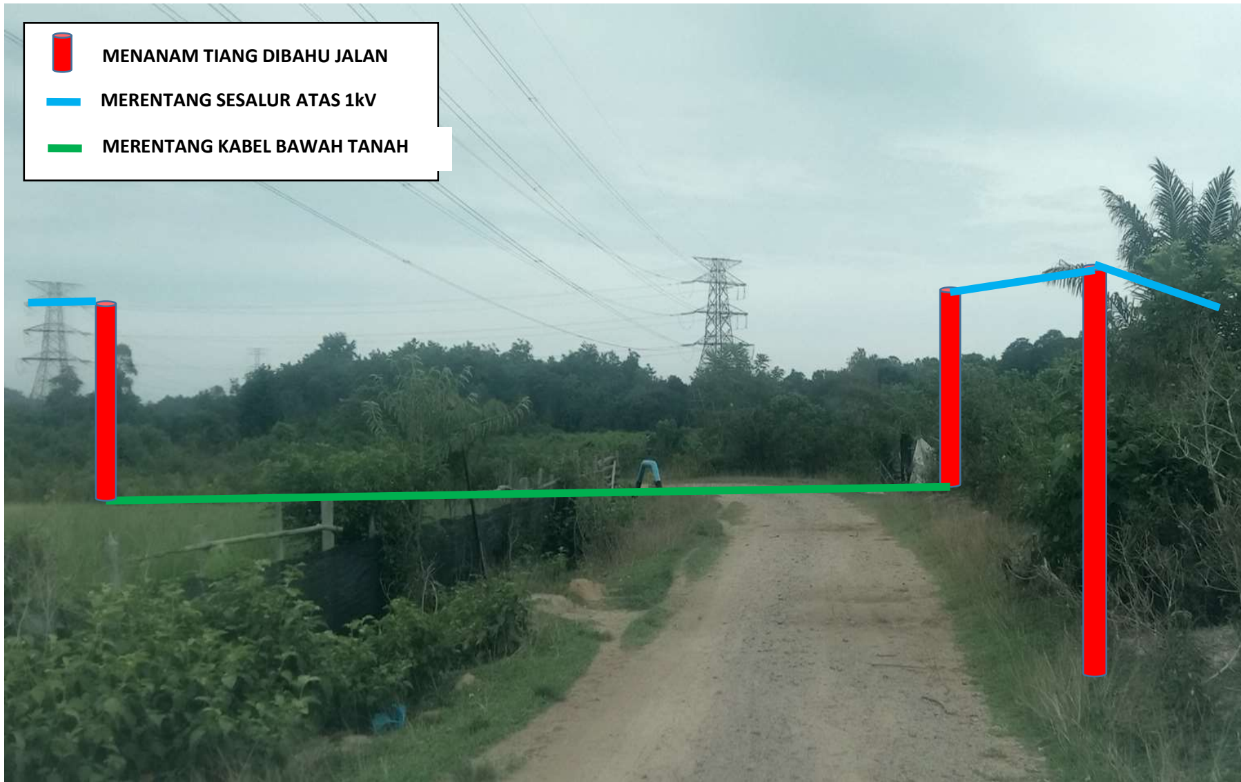
GAMBAR 5 : KAWASAN KERJA MENANAM TIANG 9.0M(2.0kN), RENTANGAN SAVR BARU DAN RENTANGAN KABEL BAWAH TANAH. (PELAN MSVR_2)
