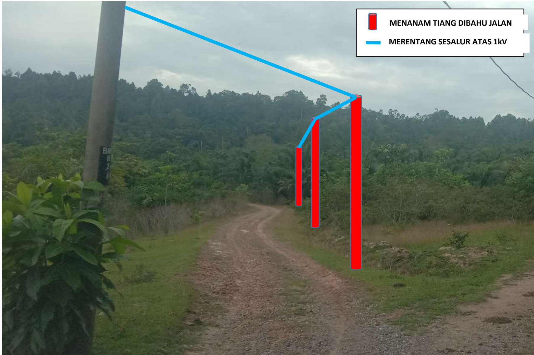
GAMBAR 1 : PERMULAAN KAWASAN KERJA MENANAM TIANG 9.0M(2.0kN) DAN RENTANGAN SAVR BARU. (PELAN MSVR_1)
