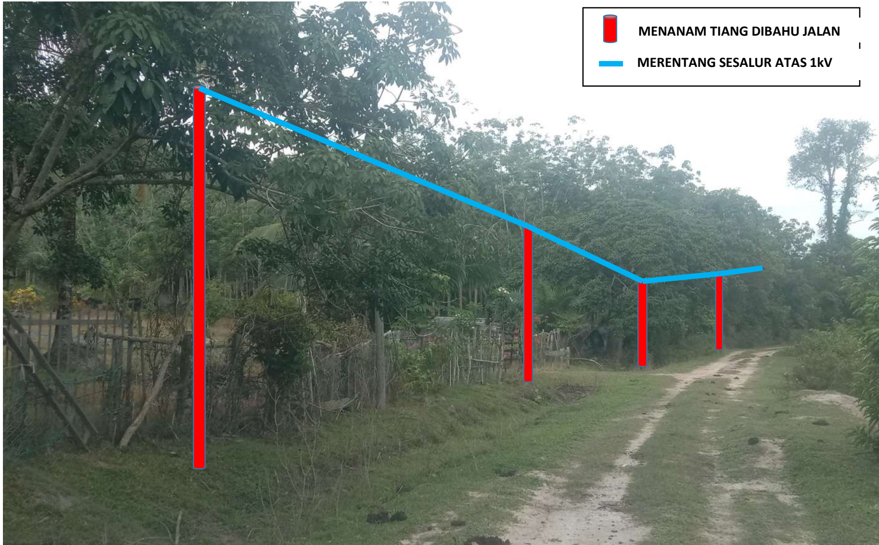
GAMBAR 2 : PENGAKHIRAN KAWASAN KERJA MENANAM TIANG 9.0M(2.0kN) DAN RENTANGAN SAVR BARU. (PELAN MSVR_1)
