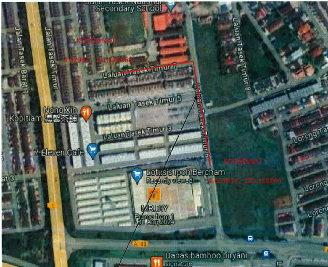
Cadangan Saluran Pembentungan 225mm Diameter V.C. Pipe Sepanjang 410 meter
