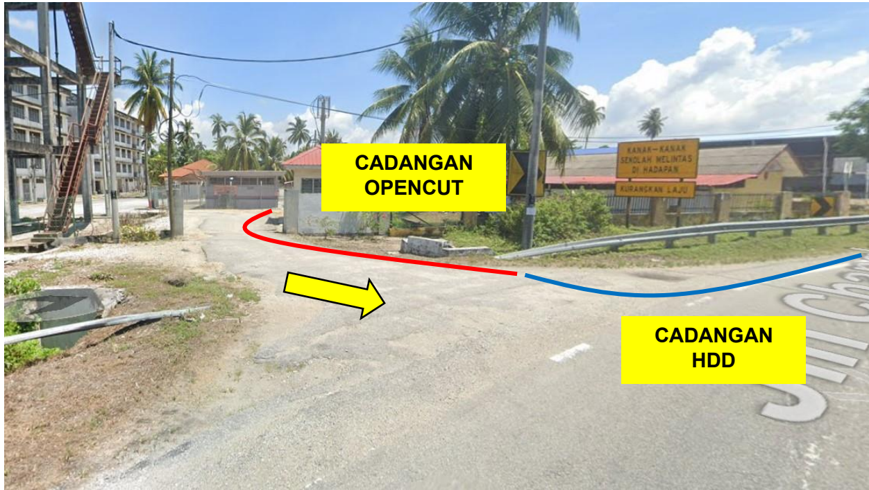
GAMBAR 1: KAWASAN KERJA MELIBATKAN PEMOTONGAN JALAN (OPEN CUT) DAN 'HORIZONTAL DIRECTIONAL DRILLING'
