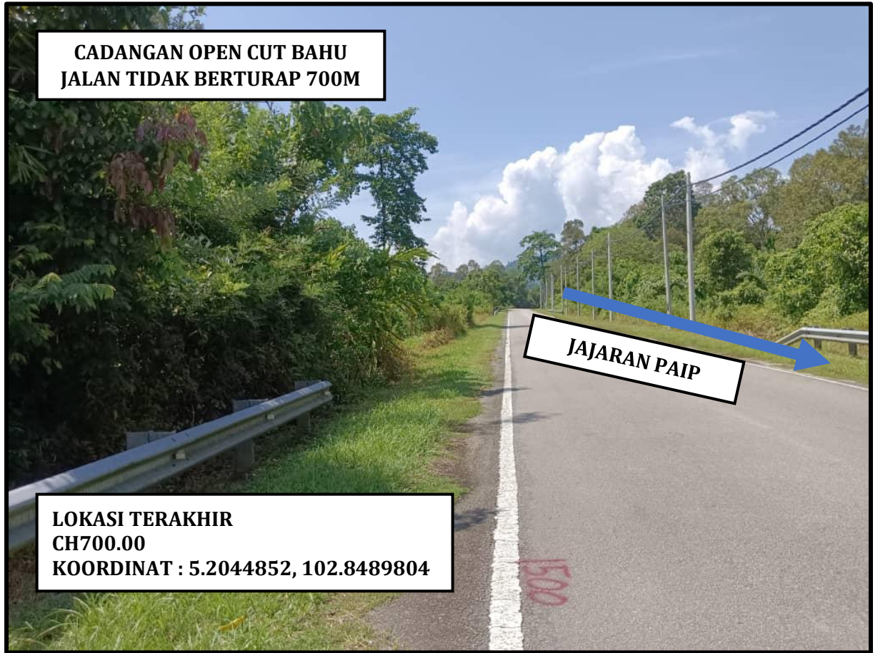
GAMBAR 3 : CH TERAKHIR KERJA PENGGALIAN BAHU JALAN TIDAK BERTURAP
