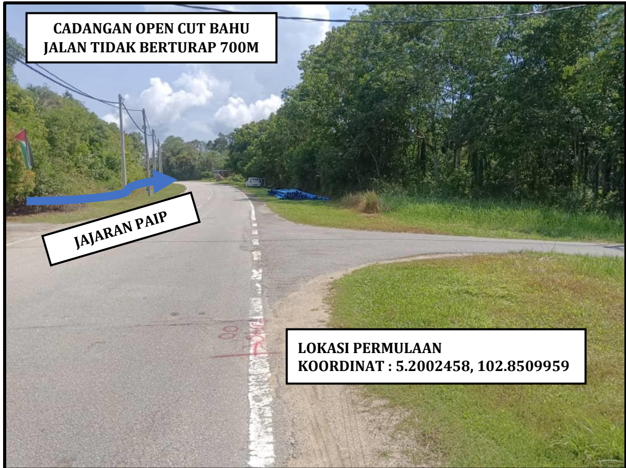
GAMBAR 2 : PERMULAAN KERJA PENGGALIAN BAHU JALAN TIDAK BERTURAP
