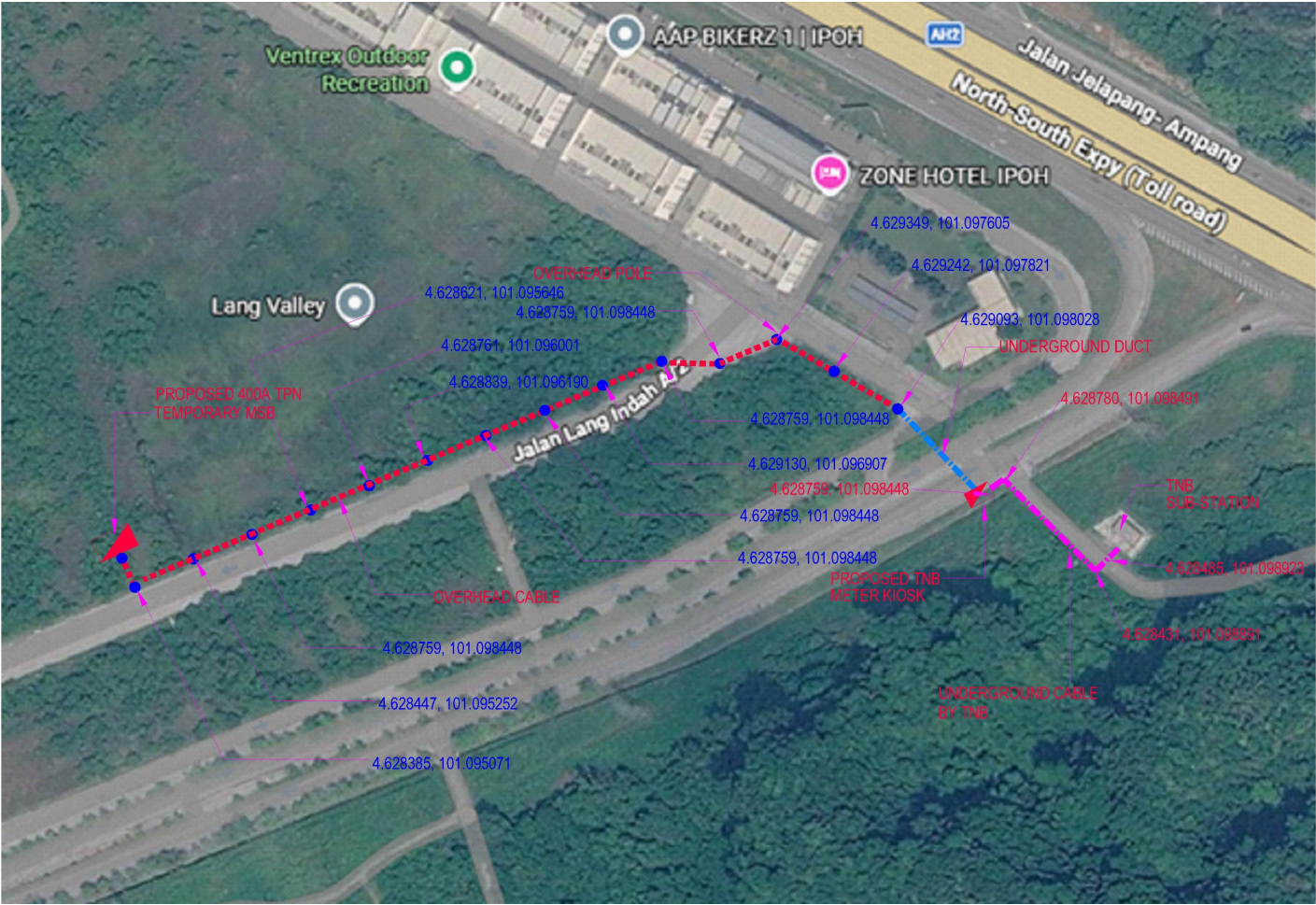
GAMBAR TAPAK
