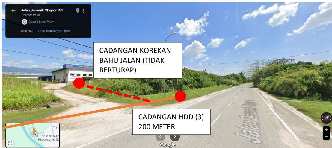
GAMBAR 9: KAWASAN KERJA MELIBATKAN 'HORIZONTAL DIRECTIONAL DRILLING' & PEMOTONGAN BAHU JALAN (TIDAK BERTURAP)
