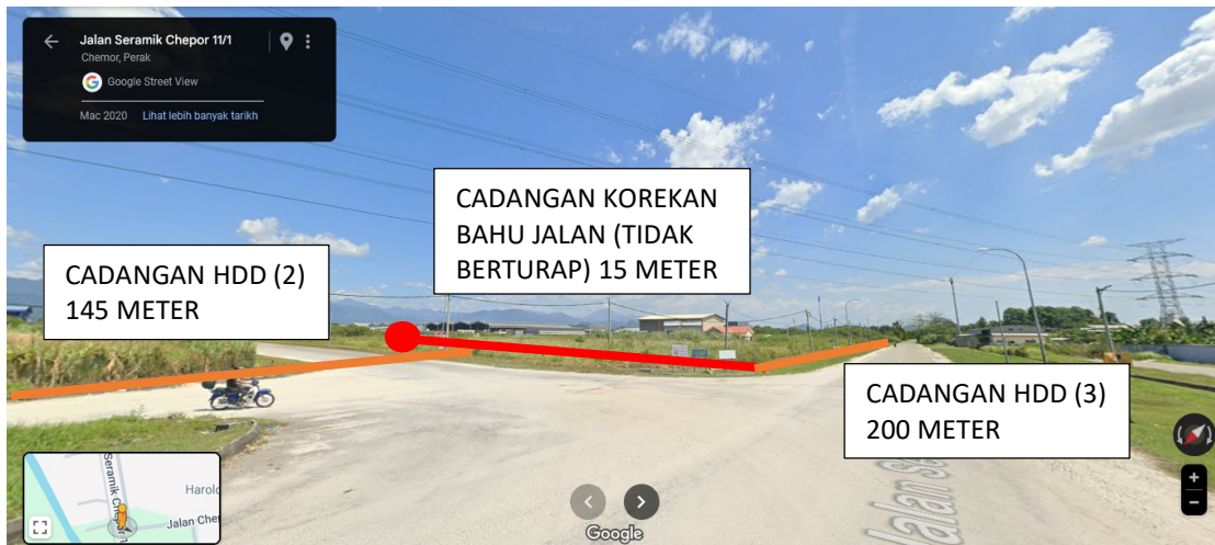
GAMBAR 5: KAWASAN KERJA MELIBATKAN 'HORIZONTAL DIRECTIONAL DRILLING' & PEMOTONGAN BAHU JALAN (TIDAK BERTURAP)
